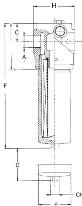
Fig. 3: También disponible en conexión SAE 1 1/4 6000 a pedido
