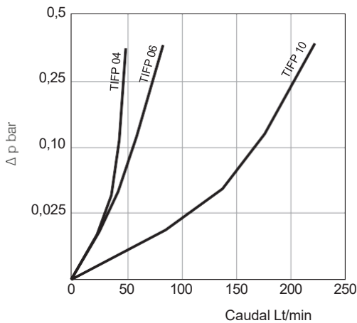
Caida de presión con aceite 36 CST@40°C con elemento de papel de 10 µm
