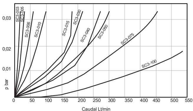
Caida de presión de aceite 36 St@ 40°C
