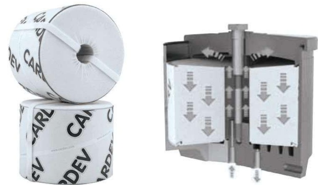
Diagrama de funcionamiento del elemento filtrante CARDEV SDFC.
