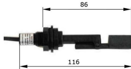
LVO N.C. sin fluido
