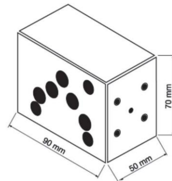
TIPO FO B10 (CETOP 5)
