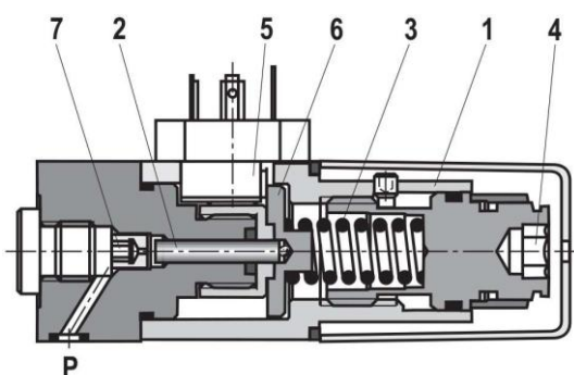
Tipo HED 8 OP-2X/...K14A Tipo HED 8 OP-2X/...K14AS
