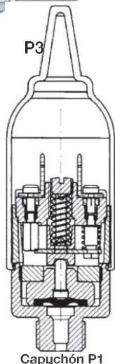
Capuchón P1
