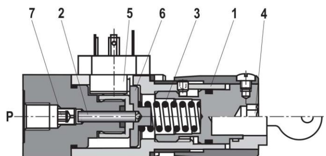
Tipo HED 8 OA-2X/...K14KW Tipo HED 8 OA-2X/...K14KS
