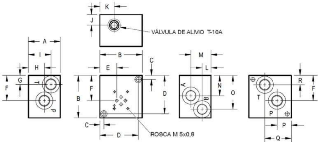
Placa base con salida dual y válvula de alivio en P Cetop 03
