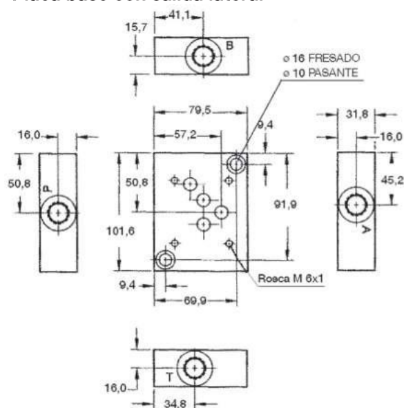
Placa base con salida lateral
