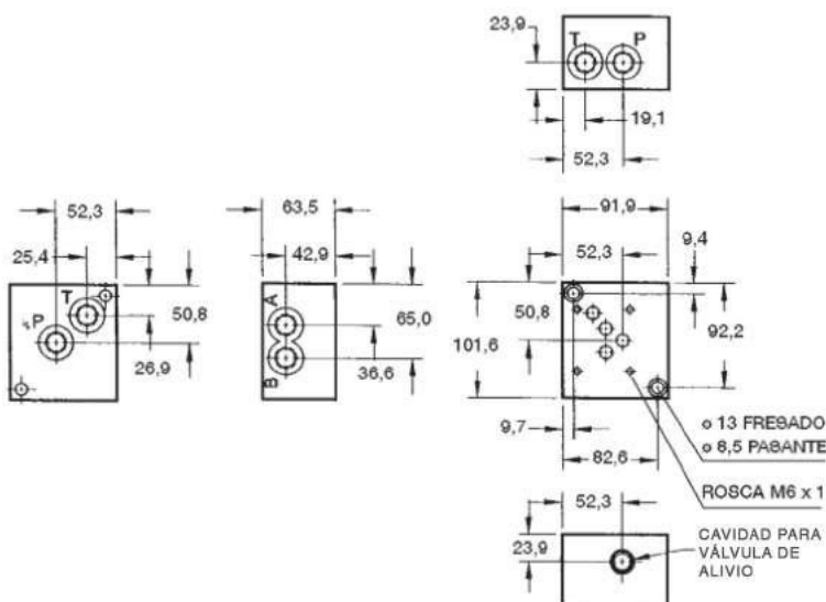
Placa base con salida dual y válvula de alivio en P Cetop 05
