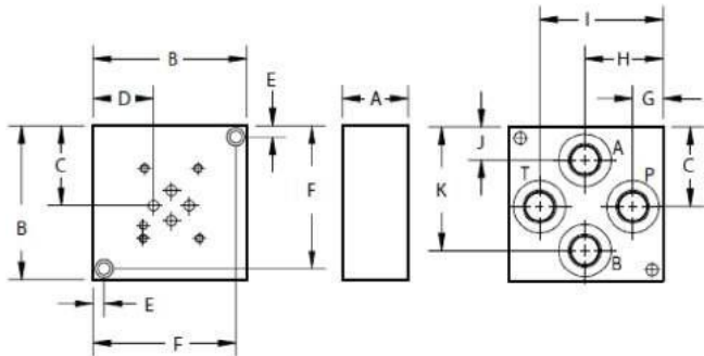
Placa base con salida inferior
