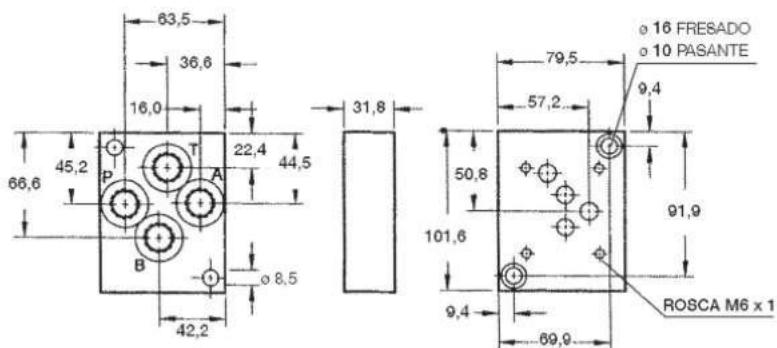
Placa base con salida inferior
