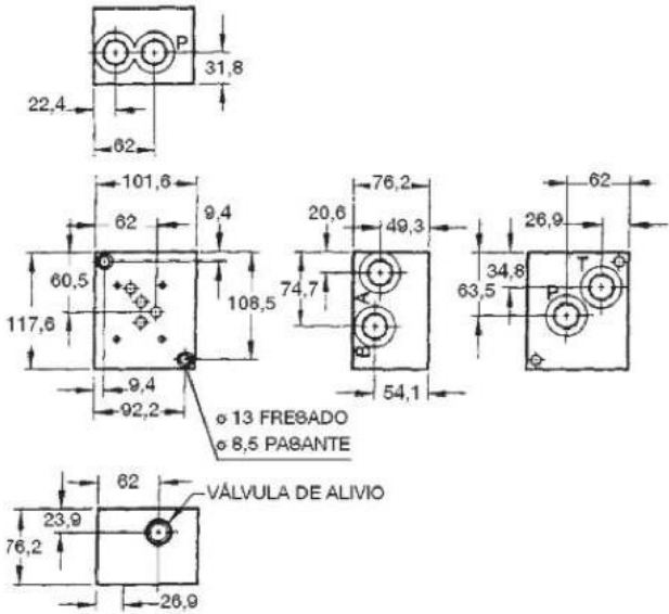
Placa base con salida dual y válvula de alivio en P Cetop 05
