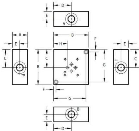
Placa base con salida lateral
