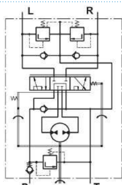
Centro abierto - No sensitivo HKUS.../4
