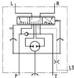
Centro cerrado - No sensitivo Señal estática - HKU.../5T
