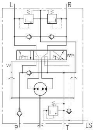
Centro cerrado - Sensitivo HKUS.../5RDT
