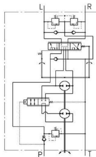
Centro abierto - No sensitivo HKUSD.../4...
