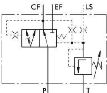
Señal dinámica PRTE 160/...
